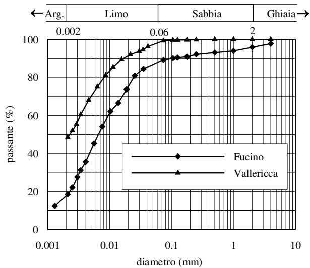
Fig. 4 – Curve granulometriche delle argille impiegate.
