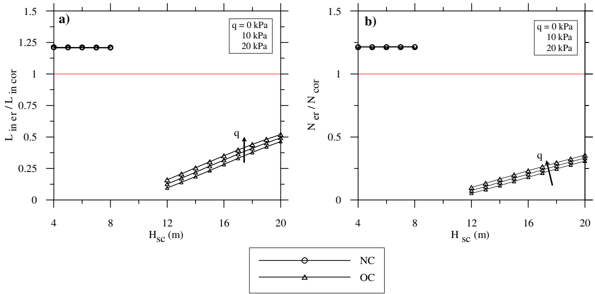
Fig. 15 – Paratia: L_{in\ er} / L_{in\ cor} e N_{er} / N_{cor} in funzione di H_{sc} . Fig. 15 – Propped retaining wall: L_{in\ er} / L_{in\ cor} and N_{er} / N_{cor} versus H_{sc} .
