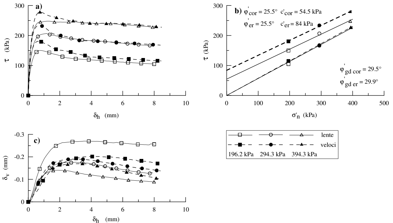
Fig. 12 – Risultati sperimentali ottenuti dalle prove di taglio sui provini OC dell’argilla del Fucino.
