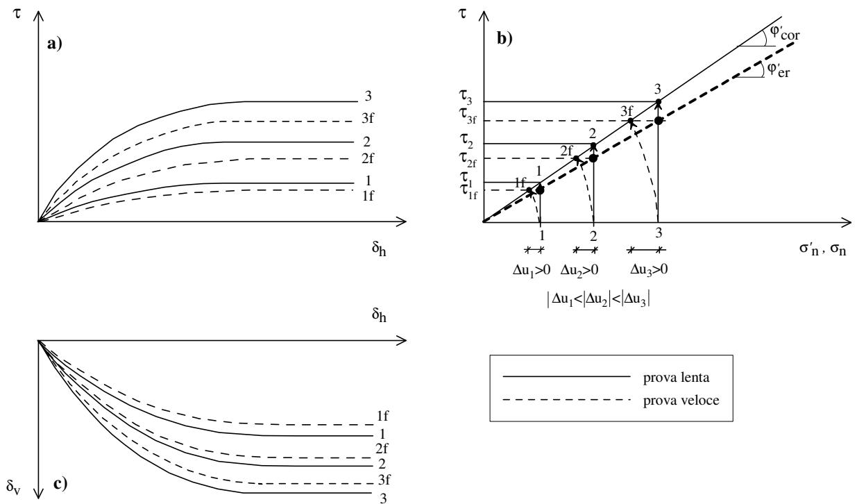
Fig. 1 – Argilla NC: evoluzione qualitativa delle tensioni normali e tangenziali sul piano di taglio.
