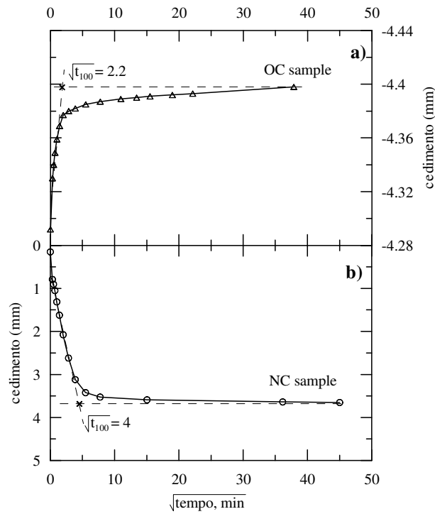
Fig. 6 – Determinazione secondo il metodo AGI del t_{100} per l'argilla di Vallericca. Fig. 6 – Evaluation of t_{100} according to AGI's method for Vallericca clay.
