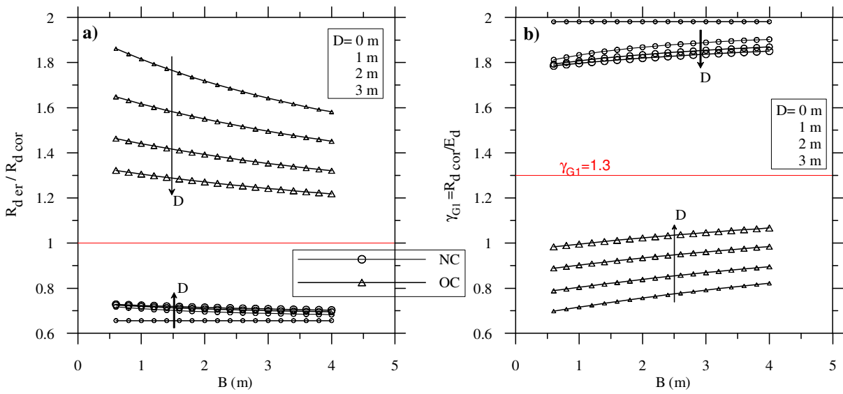
Fig. 13 – Fondazione superficiale: R_{d\ er}/R_{d\ cor} e \gamma_{GI} in funzione di B e D .
