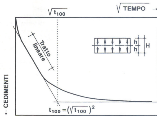
Fig. 3 – Determinazione del valore di t_{100} [AGI, 1994].
