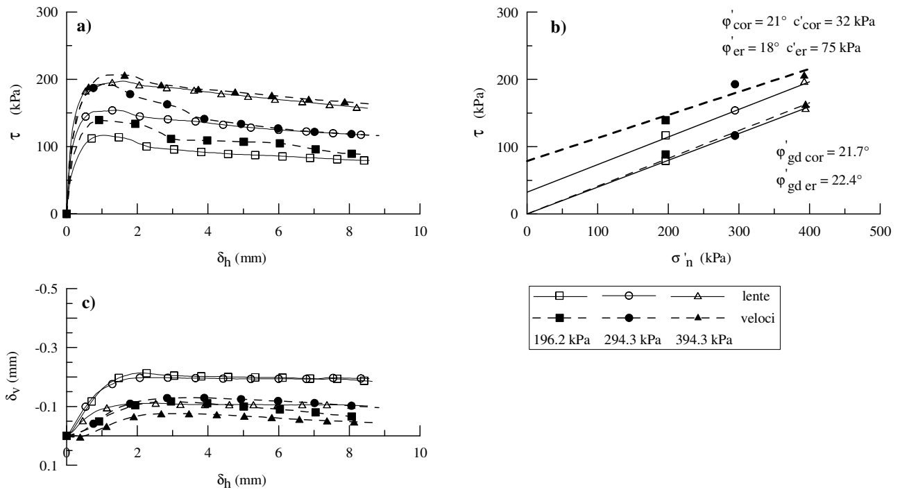
Fig. 11 – Risultati sperimentali ottenuti dalle prove di taglio sui provini OC dell’argilla di Vallericca.
